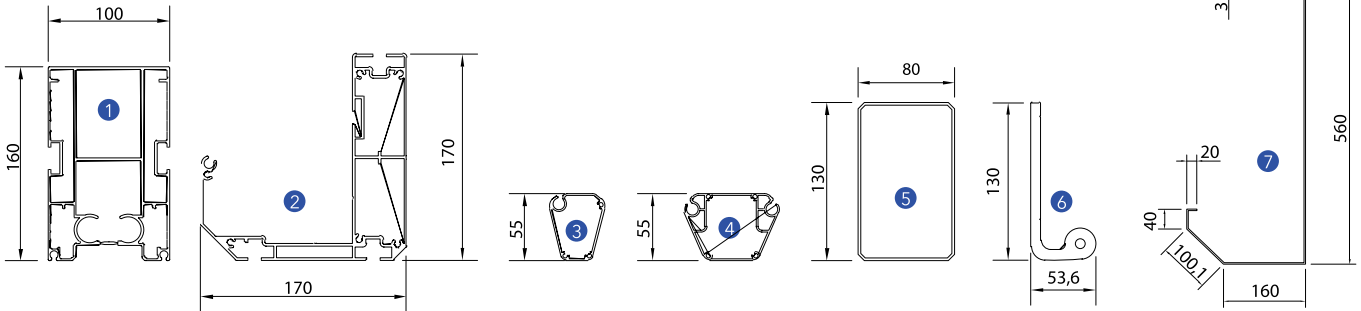
Frontal görünüş
